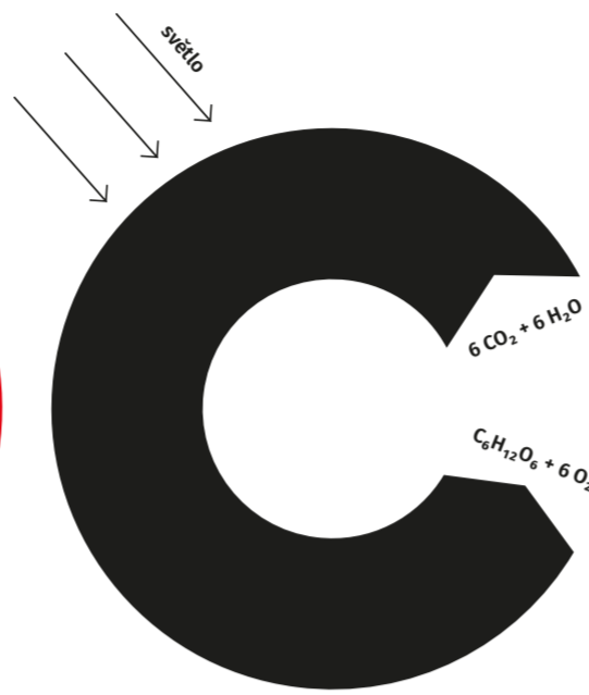
FOTOSYNTÉZA
